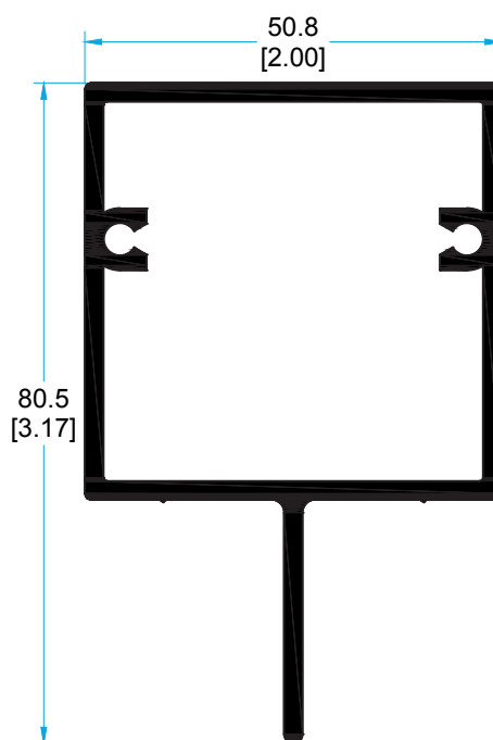
5236 INTERMEDIO LIGERO.
