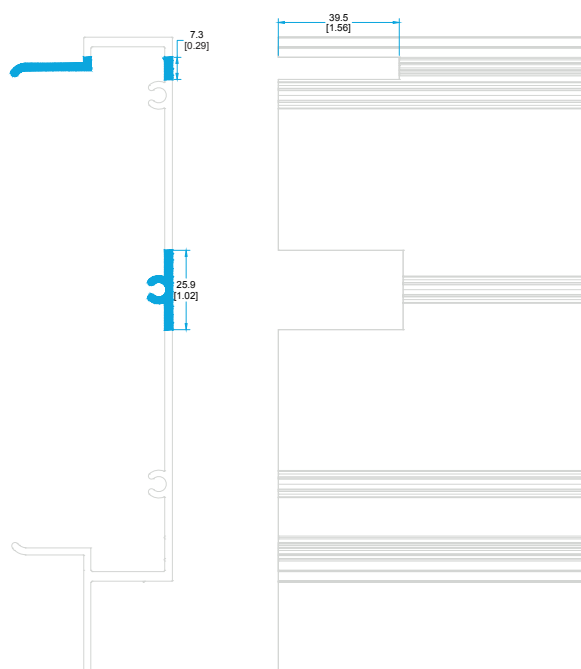
MECANIZADO PERFIL MACHO.
