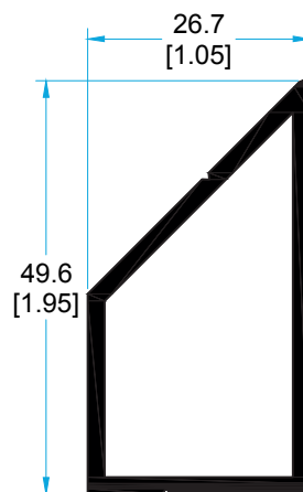
5244 ESQUINERO TUBULAR.
