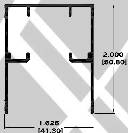
11174 RIEL
