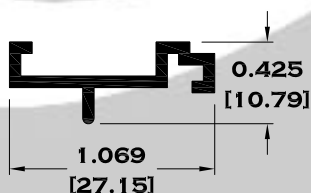
9966 ADAPTADOR MOSQUITERO
