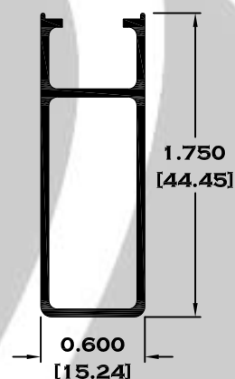
7821 CERCO PUERTA
