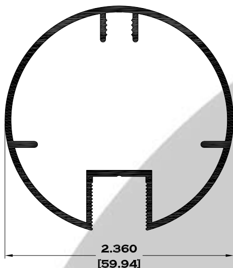
23896 PASAMANOS 2"
