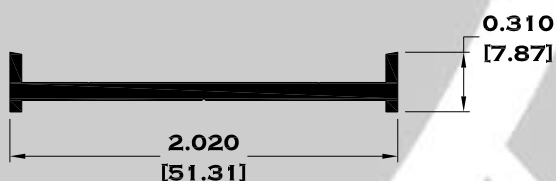
7676 SOLERA PARA PASAMANOS
