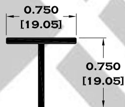
5687 TEE DE ¾"
