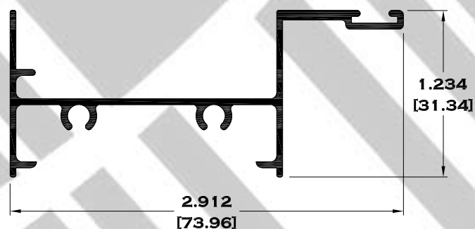
10539 JAMBA DE LUJO PARA CELOSIA
