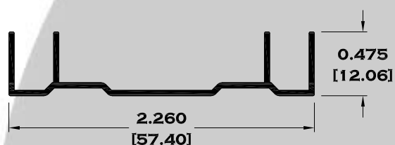
10538 CLIP PARA CELOSIA
