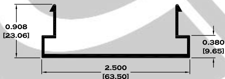
5472 TAPA BASICO ABIERTO
