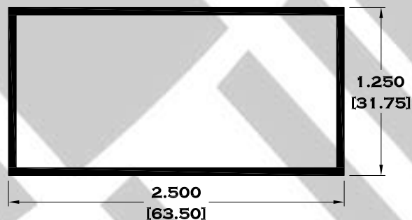
11099 TUBO RECTANGULAR DE 2 ½" X 1 ¼"
