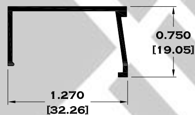
9112 JUNQUILLO
