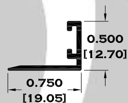
11032 BATIENTE
