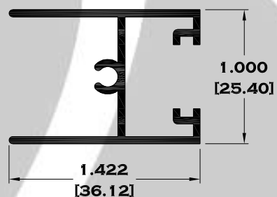
7836 CABEZAL
