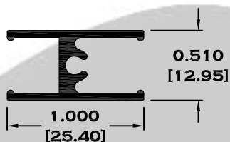
11203 INTERMEDIO PARA CUADRICULA
