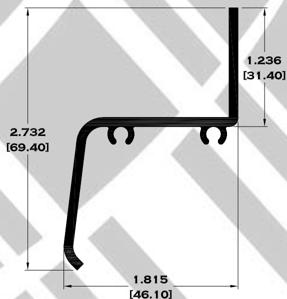
6063 LOUVER ESPECIAL
