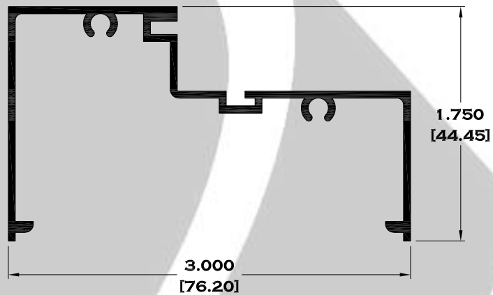
9136 ESCALONADO
