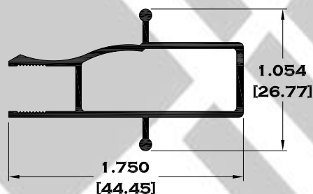
9756-B MARCO CON JALADERA
