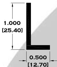
1360 ANGULO DE 1" X ½"
