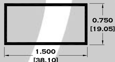
11086 TUBO RECTANGULAR DE 1 ½" X ¾"
