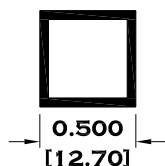
2350 TUBO CUADRADO DE 1/2"
