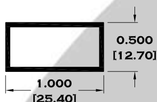
2500 TUBO RECTANGULAR DE 1" X ½"
