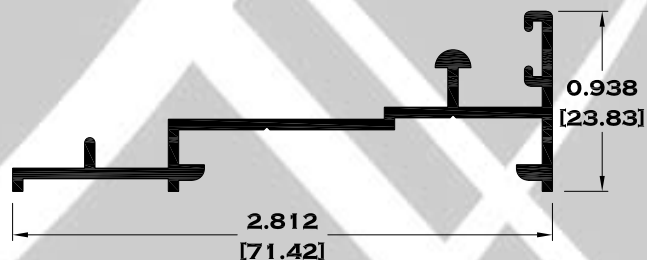
8370 RIEL DE 2" CON MOSQUITERO
