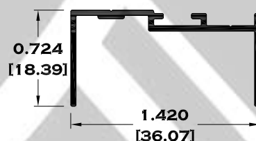
10539 JAMBA ECONOMICA PARA CELOSIA
