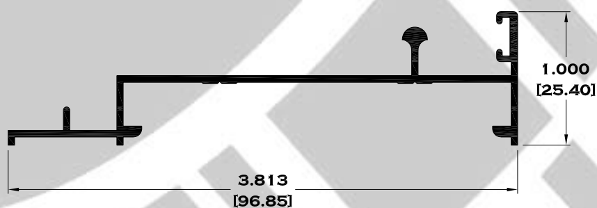
9272 RIEL CON MOSQUITERO
