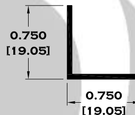
1303 ANGULO DE ¾" X 0.050"
