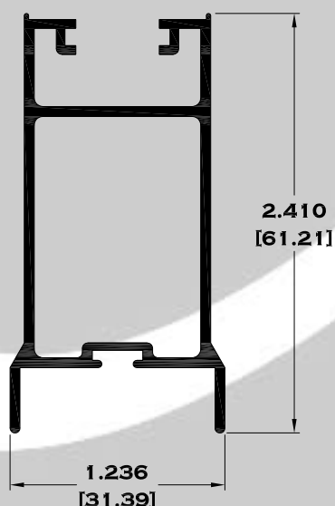
7850 CERCO OXXO
