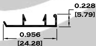
7333 LIGERO
