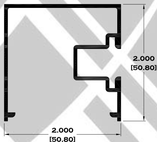
8586 ESQUINERO
