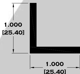
1308 ANGULO DE 1" X ⅛"
