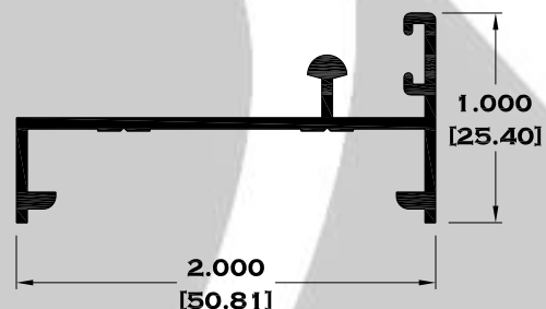
9953 RIEL
