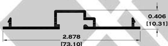
10237 TAPA BOLSA CORTA
