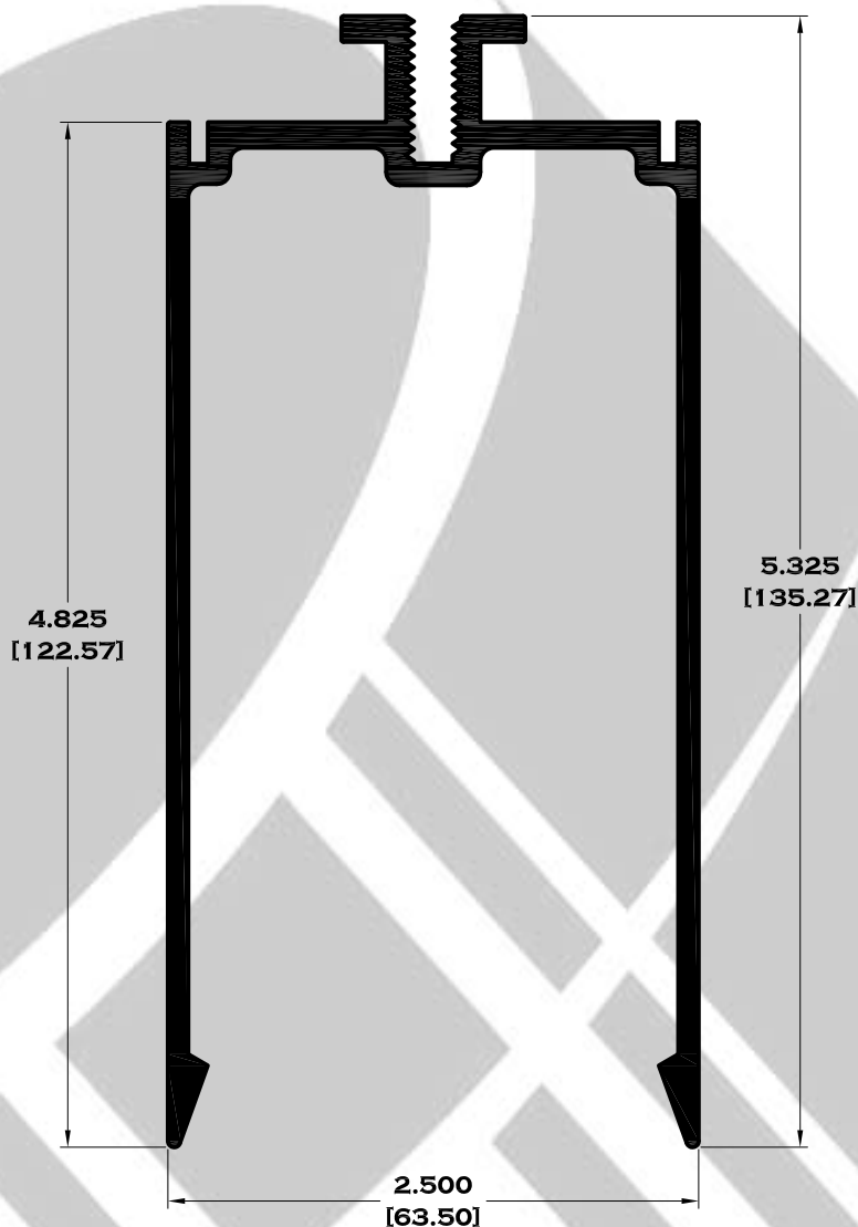
14668 BÁSICO PARA FACHADA
