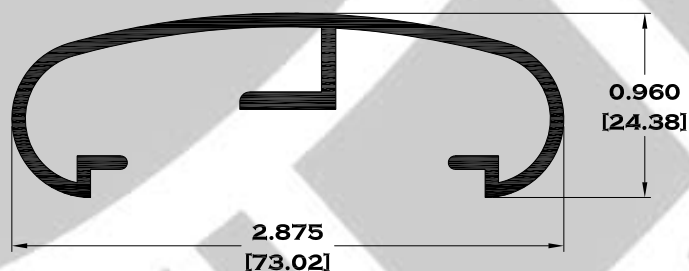
9366 PASAMANOS TIPO 002
