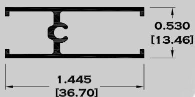
11044 ZOCLO CABEZAL
