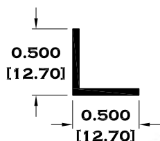
1301 ANGULO DE ½" X 0.050"
