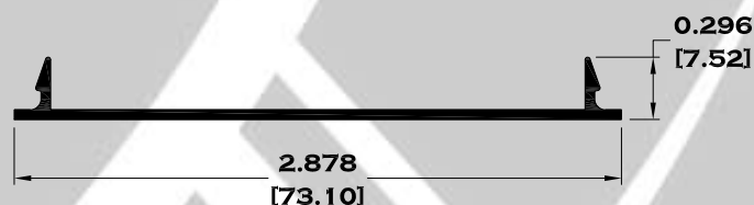
7316 TAPA LISA
