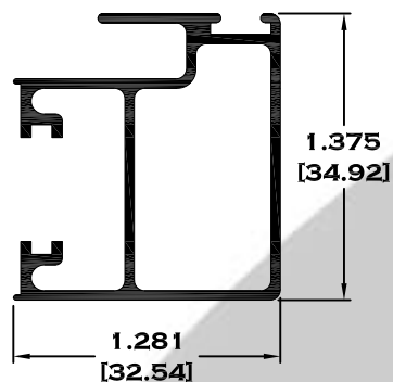
7844 TRASLAPE VENTANA
