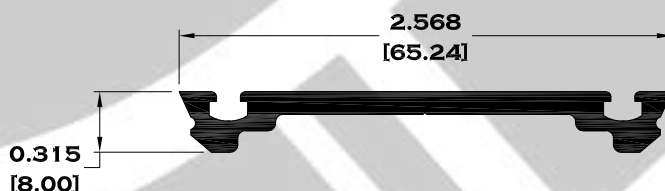
2007 PORTAVIDRIO
