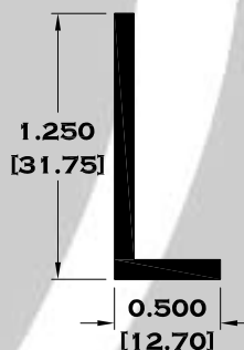
1361 ANGULO DE 1 ¼" X ½"
