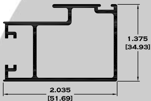
** 7848 TRASLAPE PUERTA
