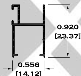
5281 CERCO TRASLAPE
