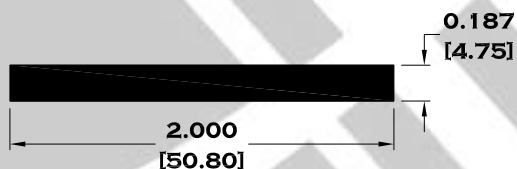
1216 SOLERA DE 2" X 3/16"
