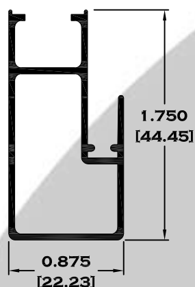
** 9955 TRASLAPE PUERTA
