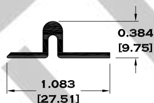
7818 RIEL ADAPTADOR
