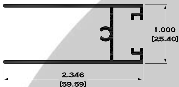
7835 ZOCLO VENTANA
