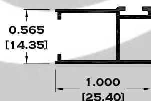
11041 CERCO TRASLAPE
