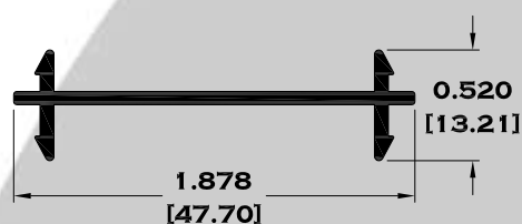
7792 MOLDURA UNIÓN 2"
