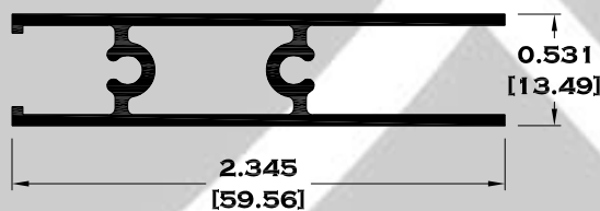
7824 ZOCLO CORTO
