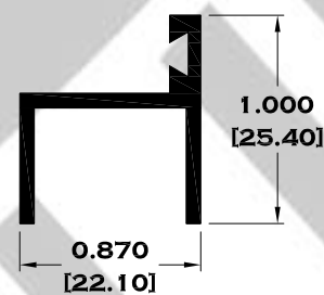
7102 BATIENTE PESADO
